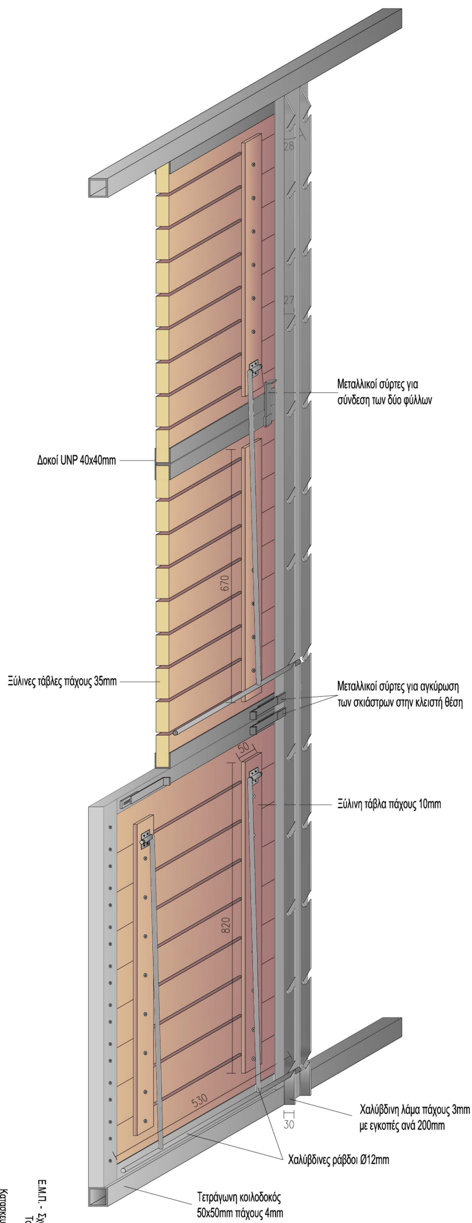
Εσωτερική όψη
