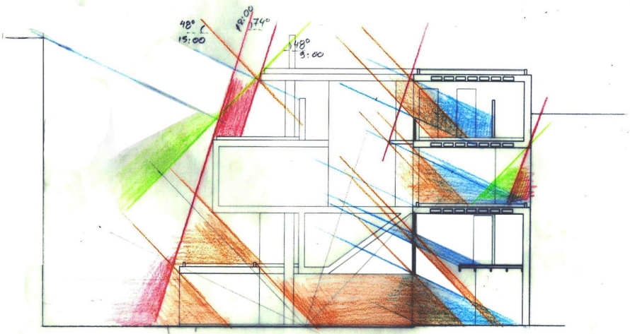
νοτιοδυτική οψοτομή
