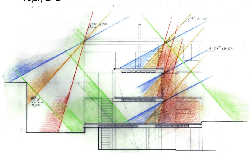
τομή B-B
