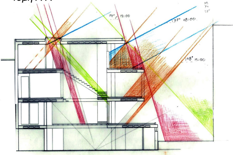
τομή A-A
