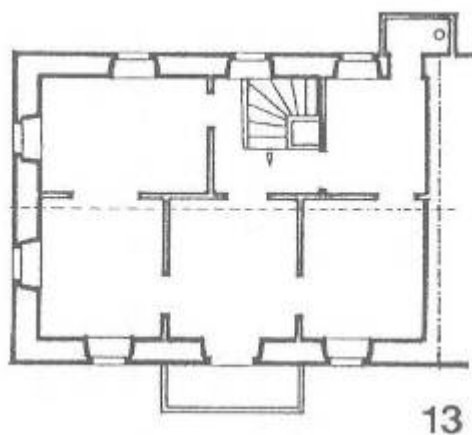
Εικόνα 13. Κάτοψη δώροφου σπιτιού - Φισκάρδο Κεφαλονιάς (πηγή: “Το ελληνικό παραδοσιακό σπίτι”, Σπ. Παπαϊωάννου, Αθήνα, 2003, πανεπιστημιακές εκδόσεις ΕΜΠ)
