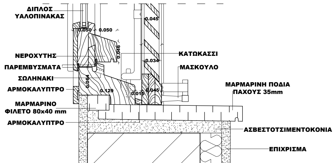
ΛΕΠΤΟΜΕΡΕΙΕΣ ΤΟΜΗΣ
