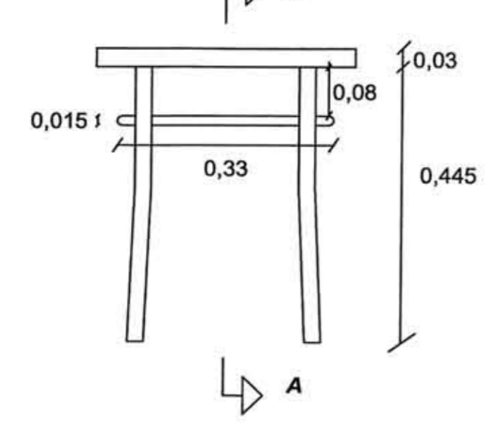
ΜΕΤΡΗΣΗ ΚΑΙ ΑΠΟΤΥΠΩΣΗ ΤΟΥ ΣΚΑΜΠΟ
