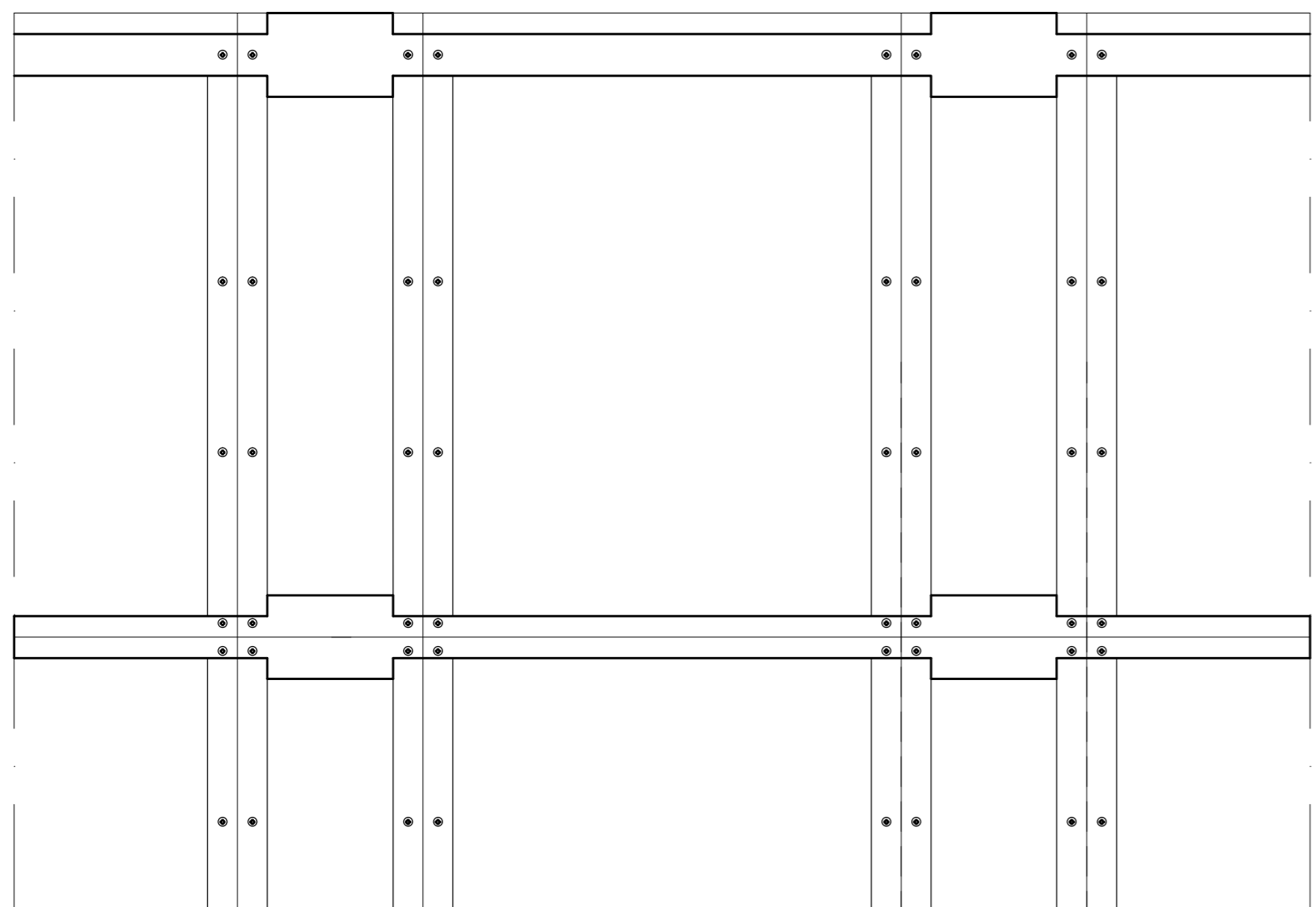
ΠΡΩΤΗ ΣΤΡΩΣΗ ΞΥΛΙΝΟΥ ΠΑΤΩΜΑΤΟΣ ΚΟΝΤΡΑ ΠΛΑΚΕ ΚΛΙΜΑΚΑ 1/10
