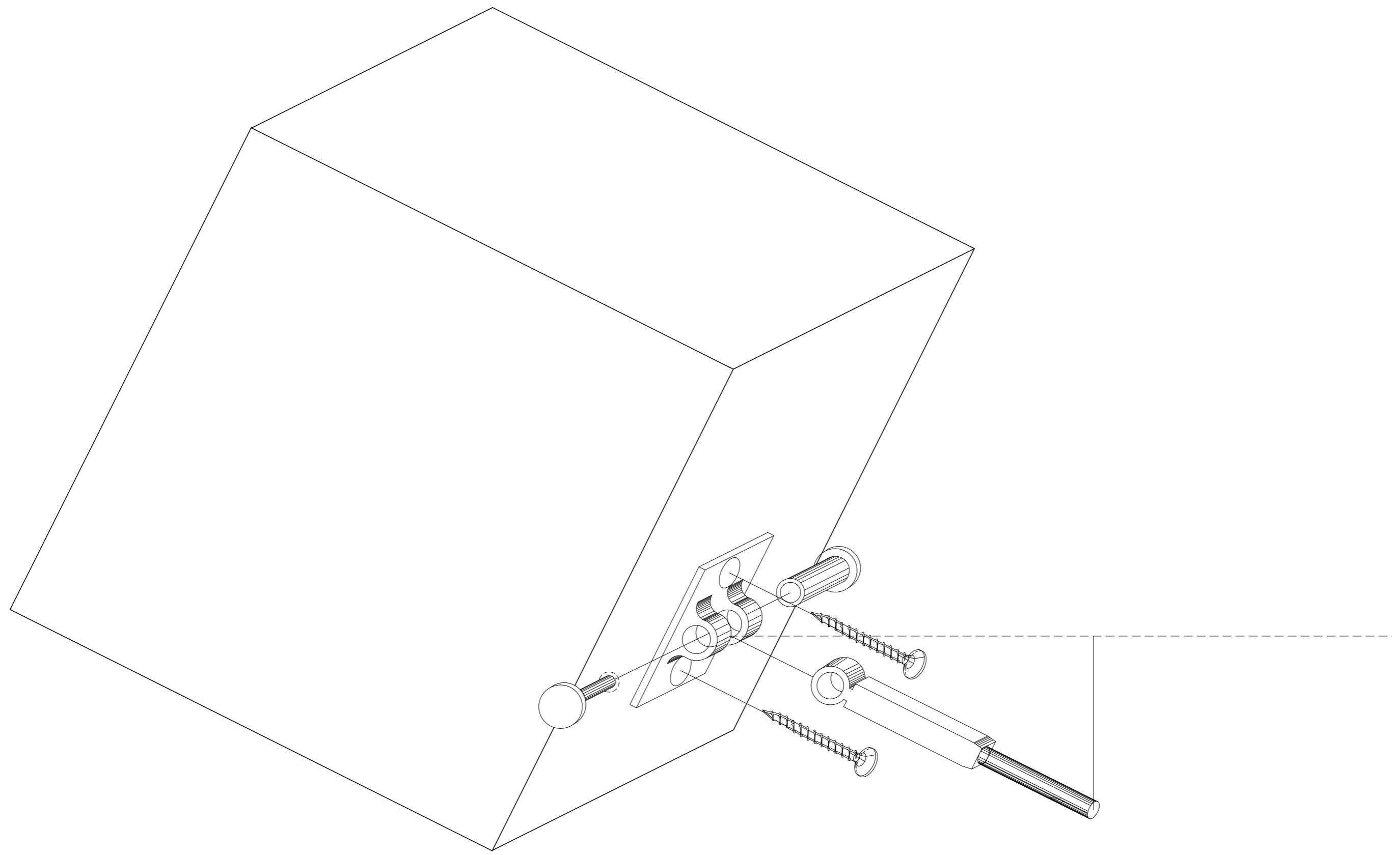
ΛΕΠΤΟΜΕΡΕΙΑ ΣΥΝΔΕΣΗΣ ΣΥΡΜΑΤΟΣΧΟΙΝΟΥ (Φ4) ΣΕ ΠΛΑΓΙΟ ΞΥΛΙΝΟ ΥΠΟΣΤΥΛΩΜΑ
