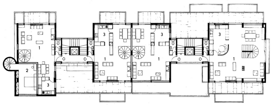
ΚΑΤΩΦΗ Δ ΟΡΟΦΟΥ
